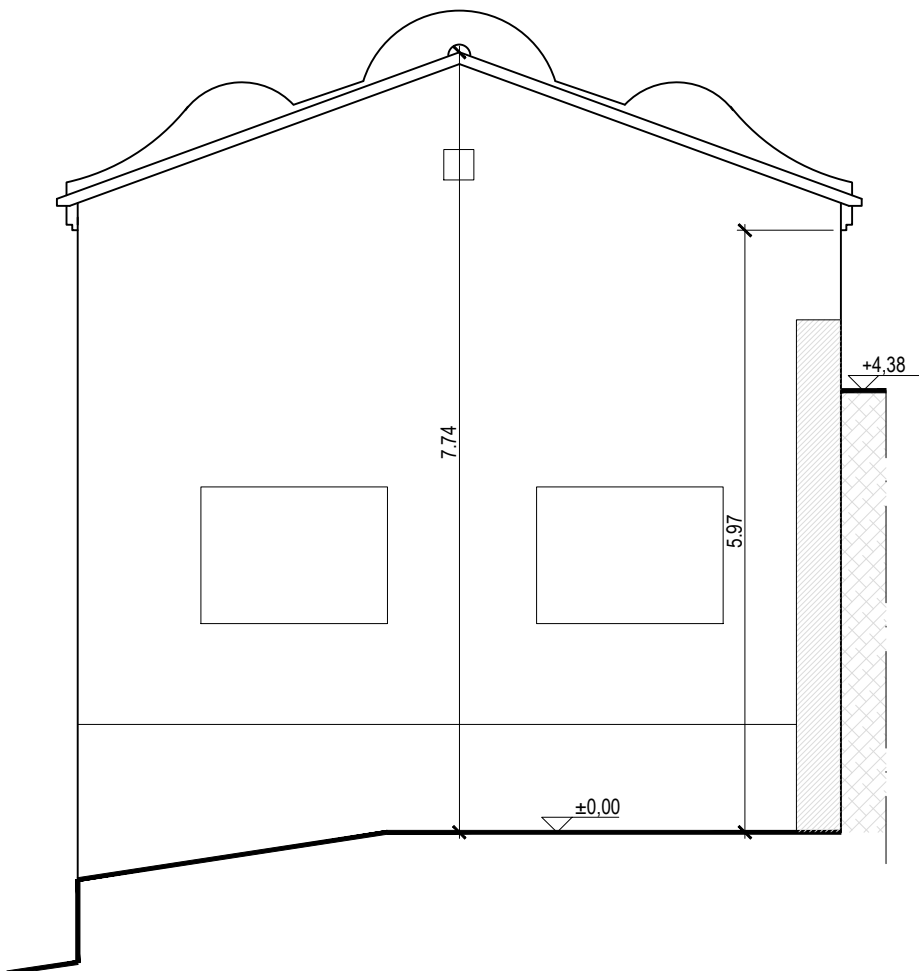
ALZADO NORESTE
