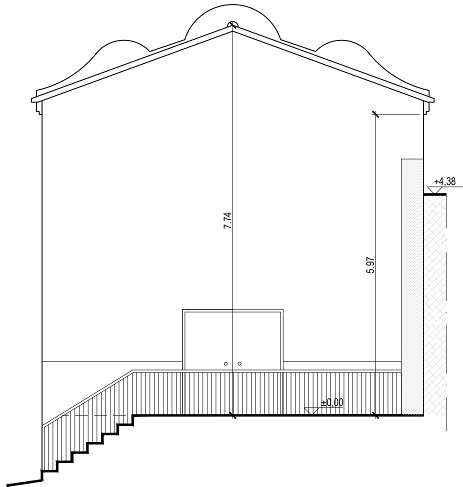
ALZADO NORESTE
