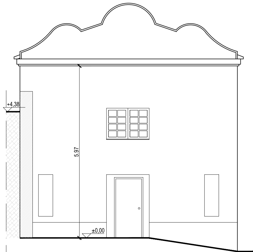
ALZADO SUROESTE
