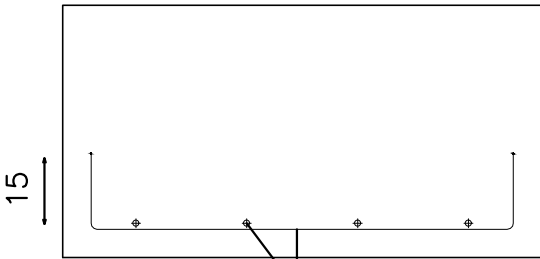
DETALLE ARMADO ZAPATAS
