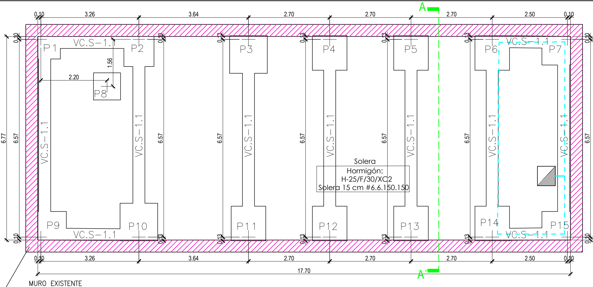
DETALLE ARMADO ZAPATAS
