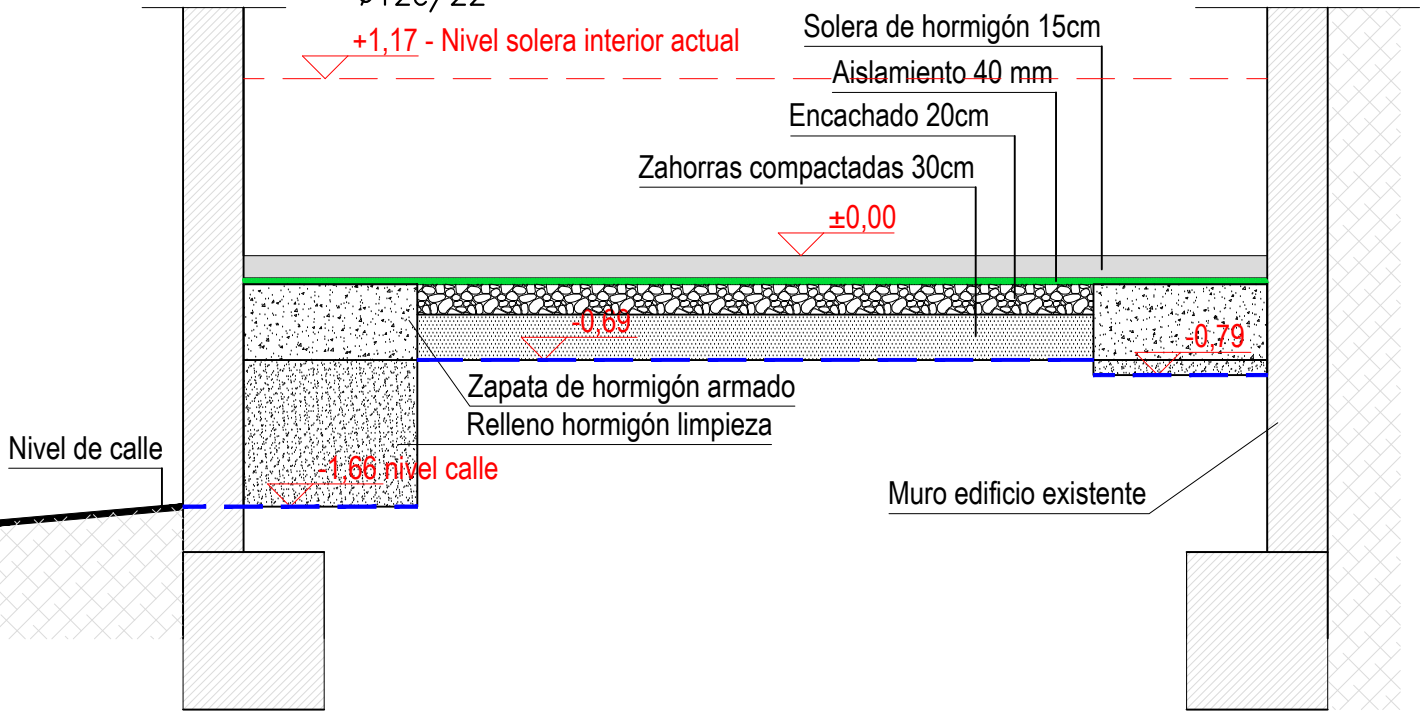
SECCIÓN A-A' E: 1/50
