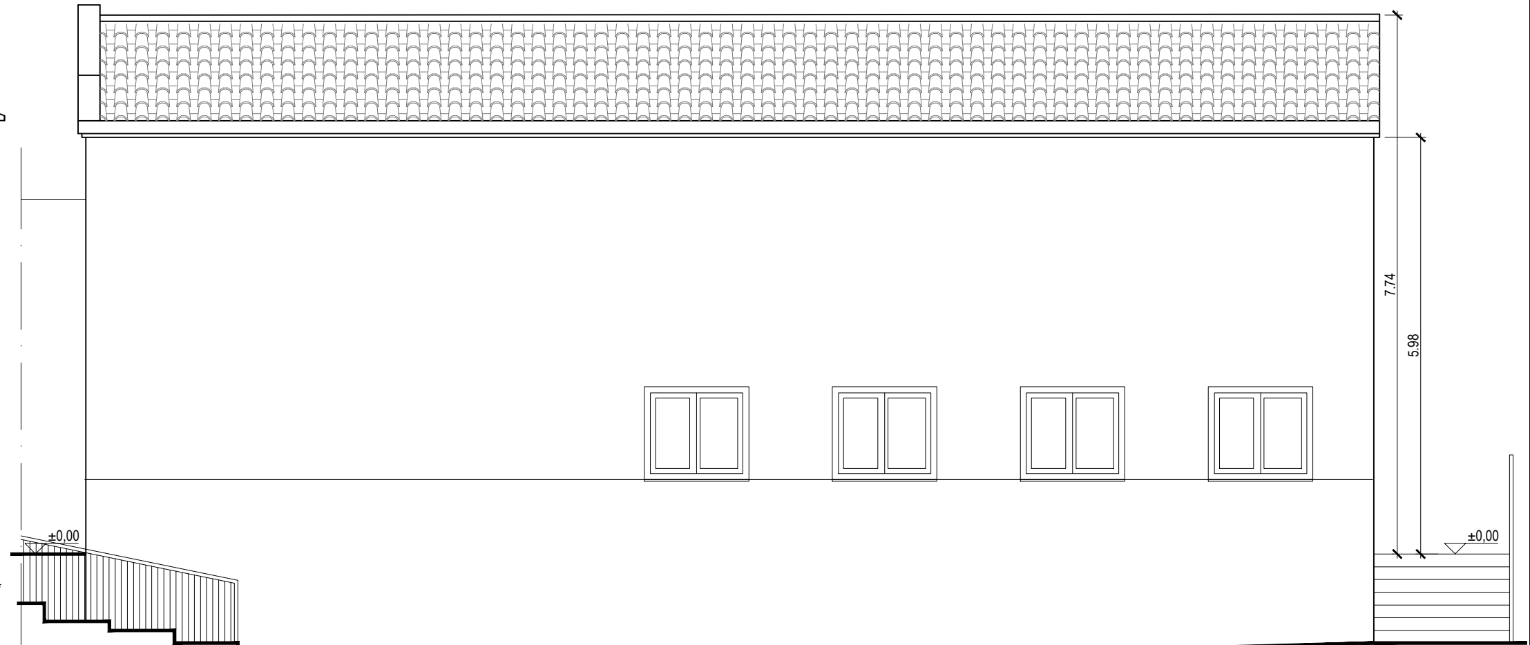
ALZADO SURESTE
