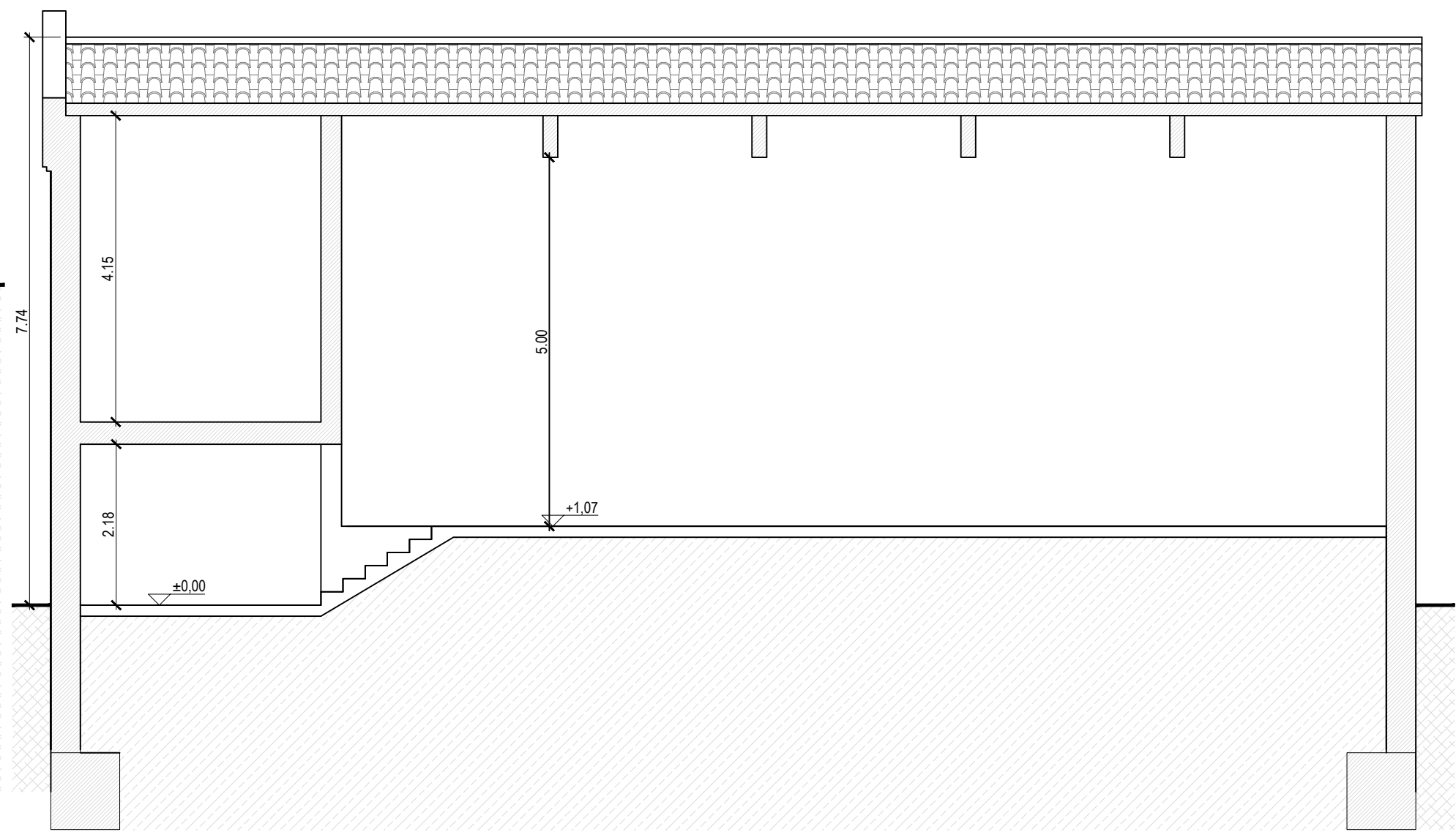
SECCIÓN B-B'
