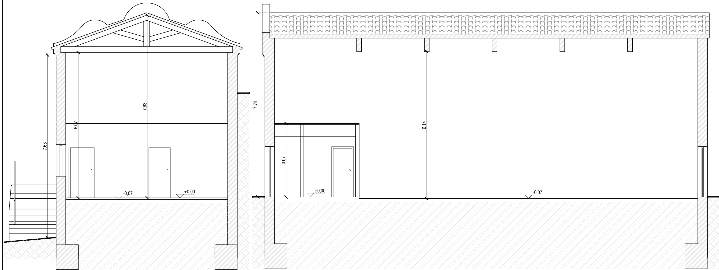
SECCIÓN A-A'
