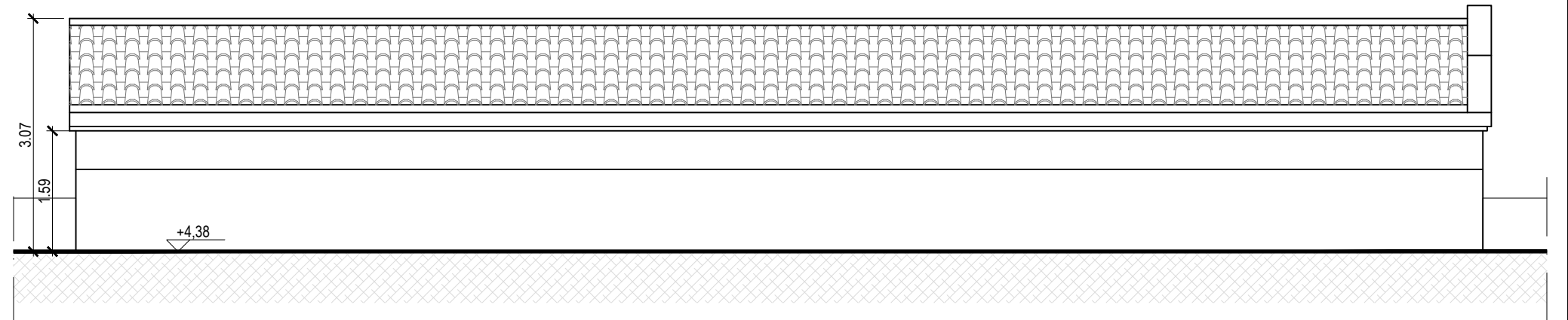
ALZADO NOROESTE
