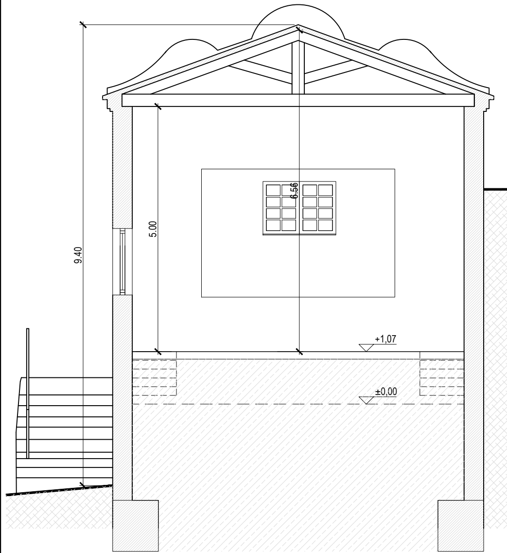
SECCIÓN A-A'
