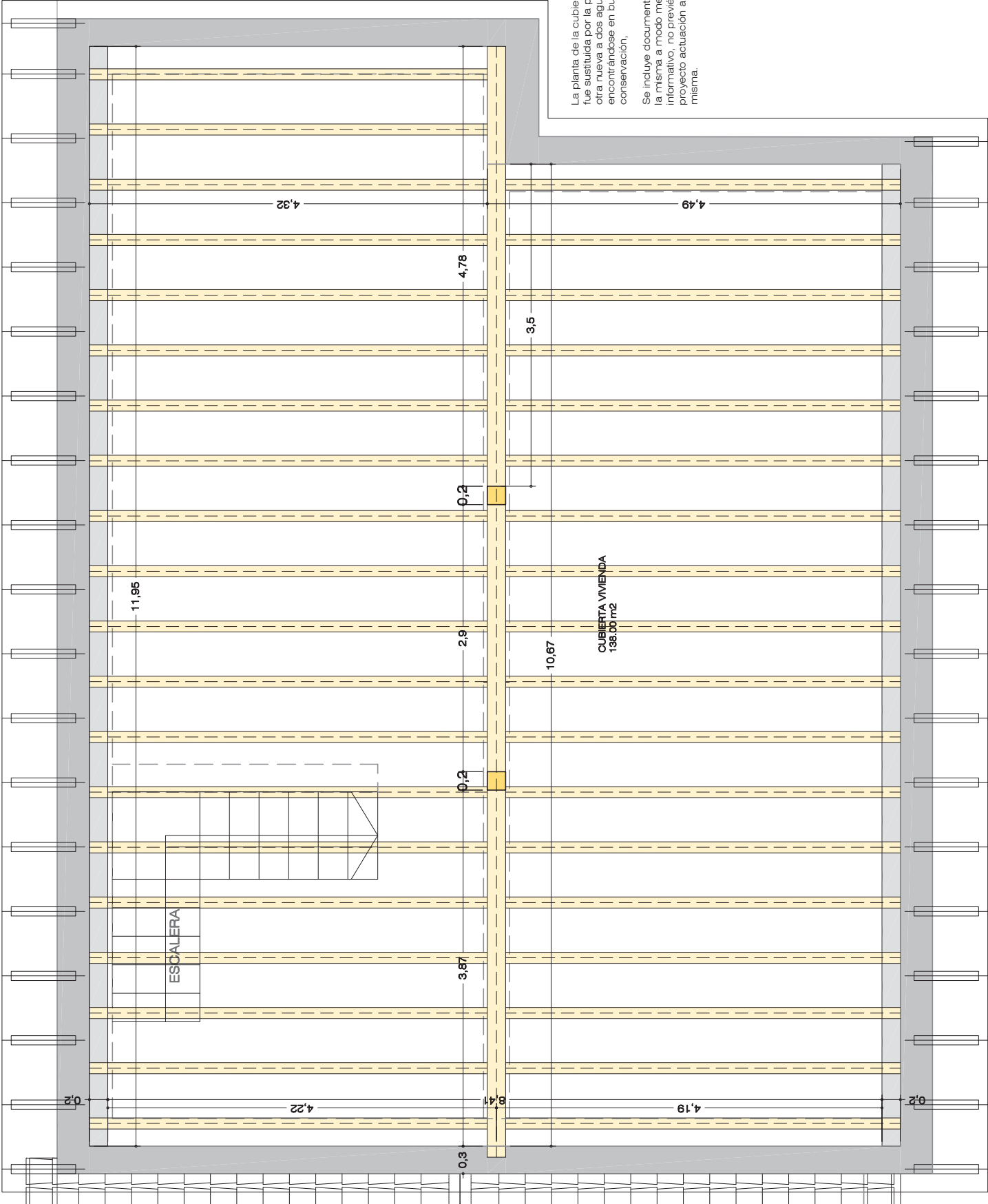
PLANTA CUBIERTA. FORJADO EXISTENTE. ESCALA 1/40
