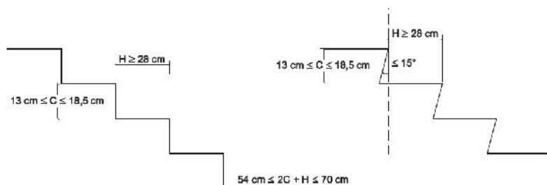
Figura 4.2 Configuración de los peldaños.
