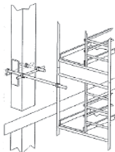
con collarín
