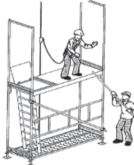
armado de andamio
